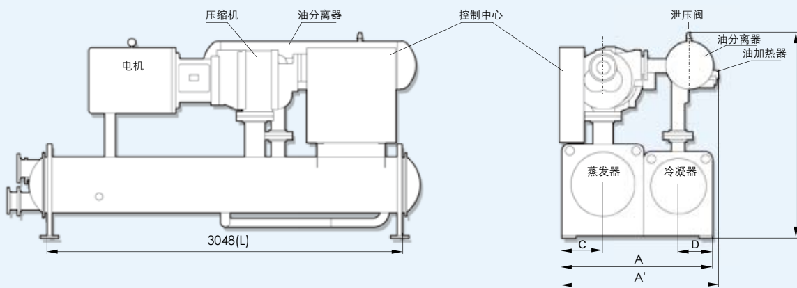
机组外型尺寸(S0-S3压缩机)
